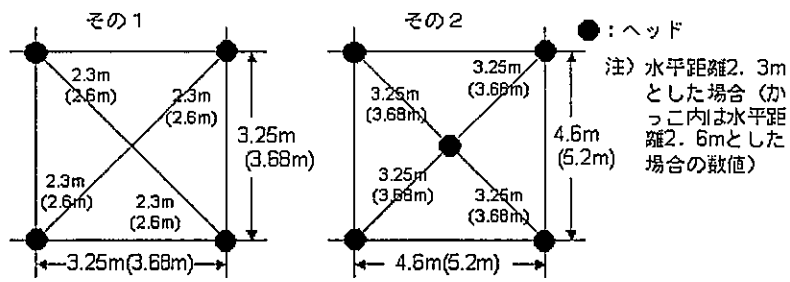
〔格子配列の例〕 第3-7図
