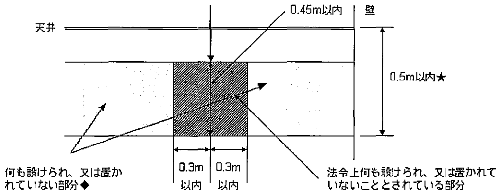
〔小区画型ヘッドの場合（特定共住省令に定める共同住宅用スプリンクラー設備に設けるものは法令基準）：断面〕
