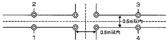
〔放水区域の重複例 ◎：放水型ヘッド〕
