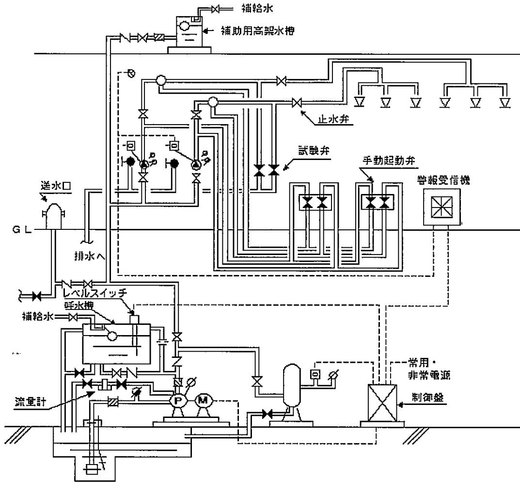
〔開放型スプリンクラー設備の配管系統例〕
