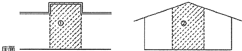
〔明かり窓、排煙等などの部分例〕
