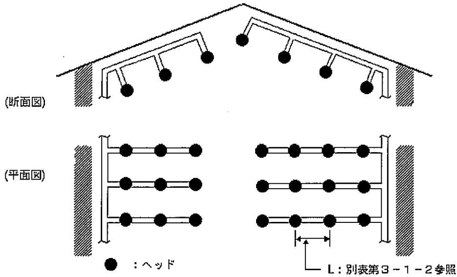
〔正方形又は矩形配置の場合の例〕
