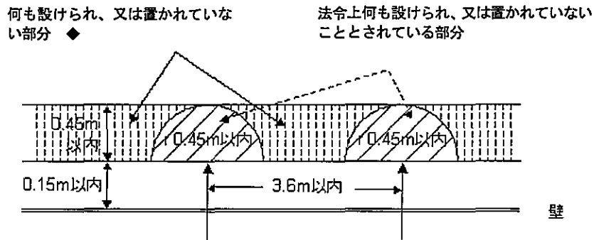
〔側壁型ヘッドの場合：平面〕
