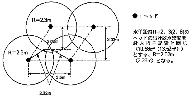
〔散水密度が低下しないようにした千鳥型配置の例〕 第3-8図
