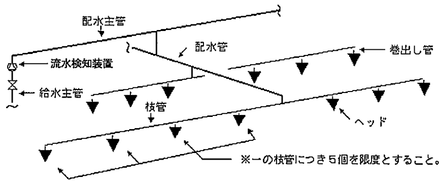
〔配管の名称及び枝管とヘッドの取付け例〕 第3-15図
